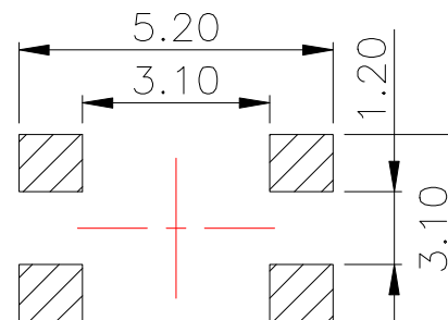
PCB.焊接图
